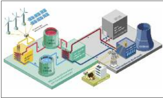
(3D-Grafik Wärmespeicher (Quelle: RWE Power))
